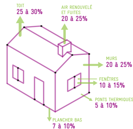
DÉPERDITIONS ÉNERGÉTIQUES D'UNE MAISON D'AVANT 1974 NON ISOLÉE
